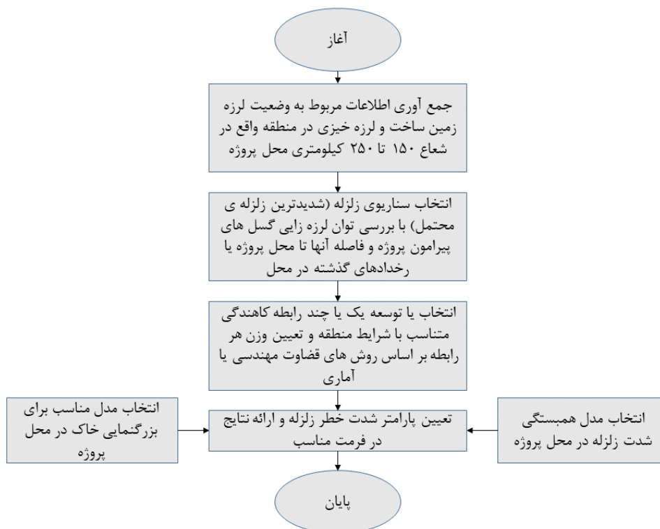
شکل ۱-۲: روندنمای مراحل لازم برای سنجش خطر زلزله به روش کمی با رویکرد تعینی (سناریومحور)
